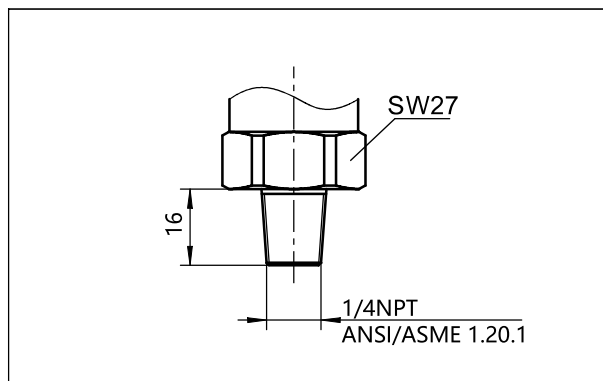
過程接続 (R02) (単位 : mm)
