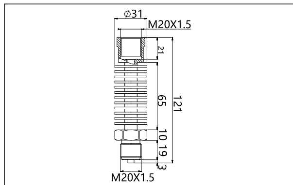
熱交換接続部品 (N2) (単位 : mm)
