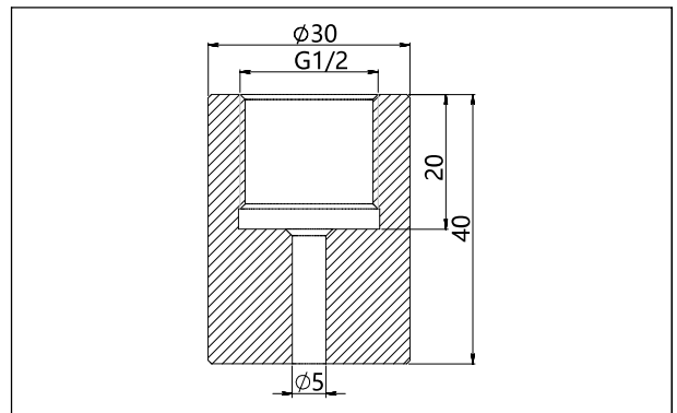
熔接伝接部品 (Z2) (単位 : mm)
