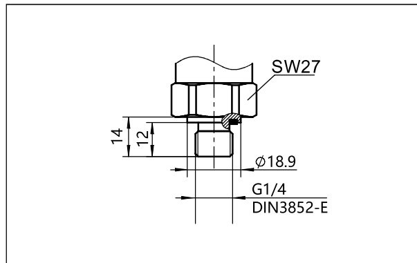
過程接続 (G08) (単位 : mm)
