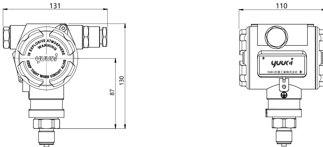
JUN-E21表示機能無し本体寸法図
