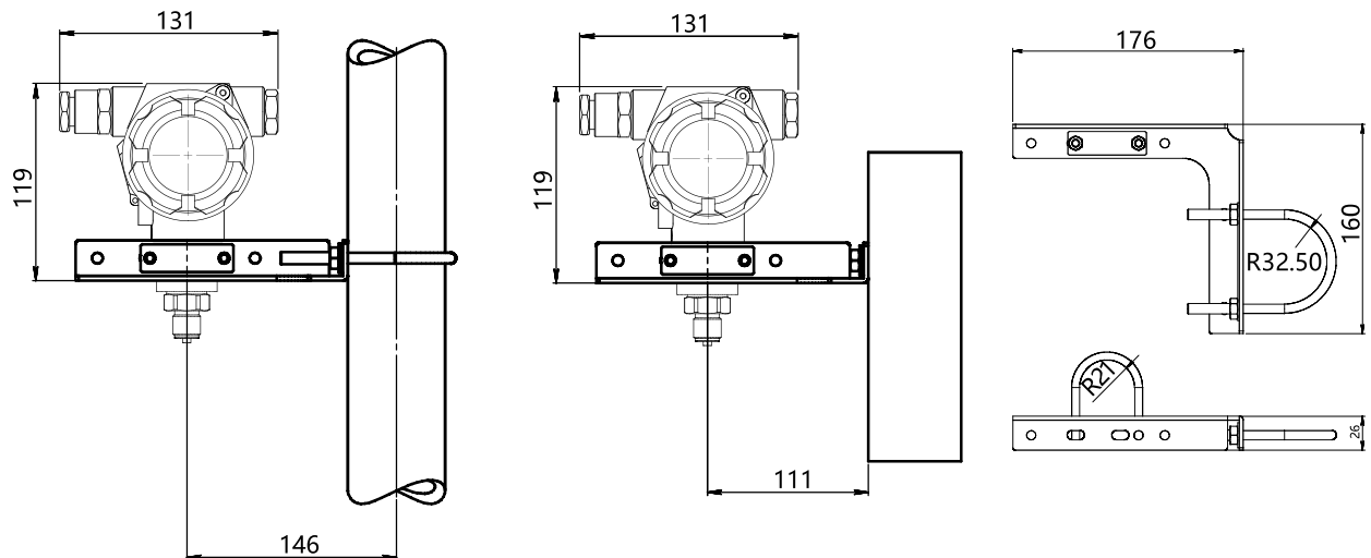
JUN-E21固定取付けスタンド(B4) 取付け寸法図
