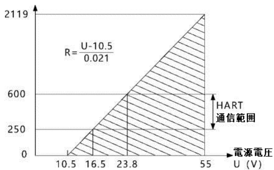
图 1 電源及び負荷条件
