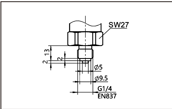
圧力導入G02寸法図
