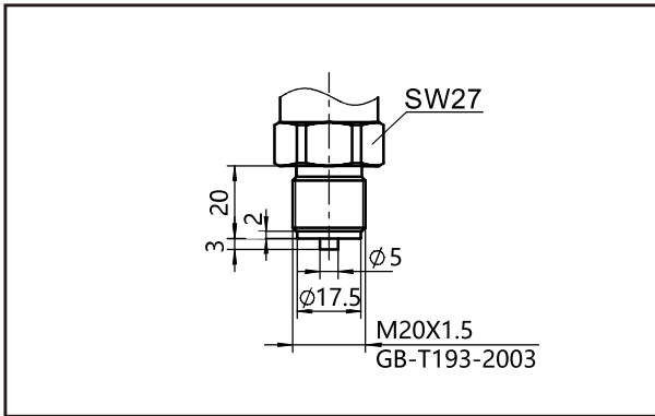
圧力導入M01寸法図
