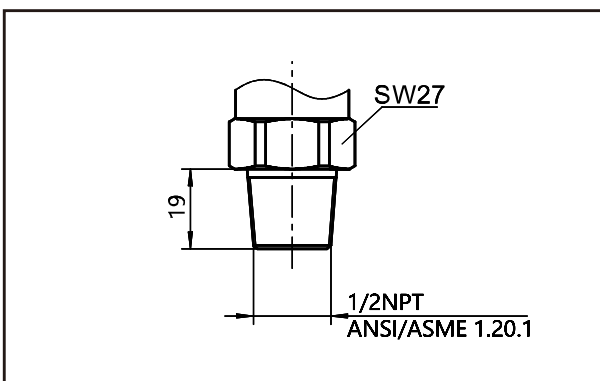
圧力導入R01寸法図
