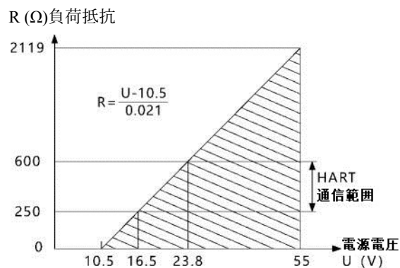
図 1 電源及び負荷条件
