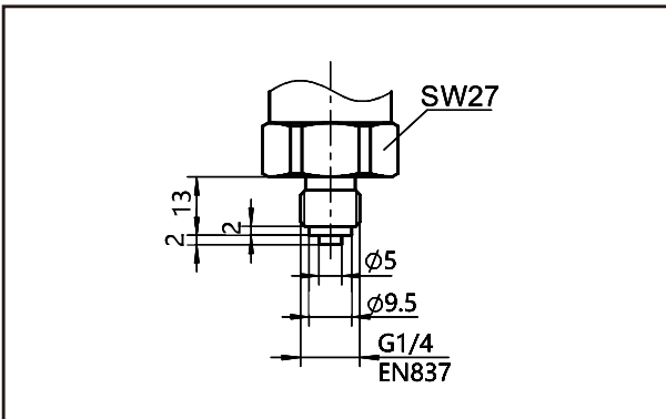
压力导入G02寸法图
