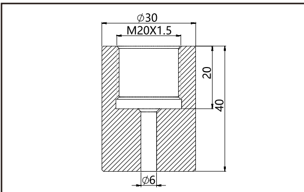
压力导入Z1寸法图
