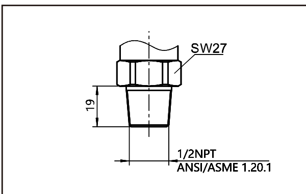
压力导入R01寸法图
