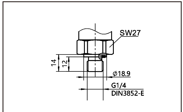
压力导入G08寸法图
