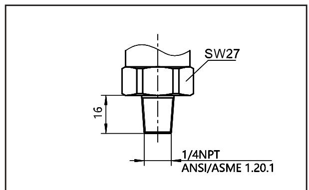
压力导入R02寸法图
