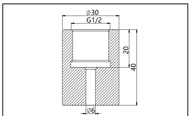
压力导入Z2寸法图
