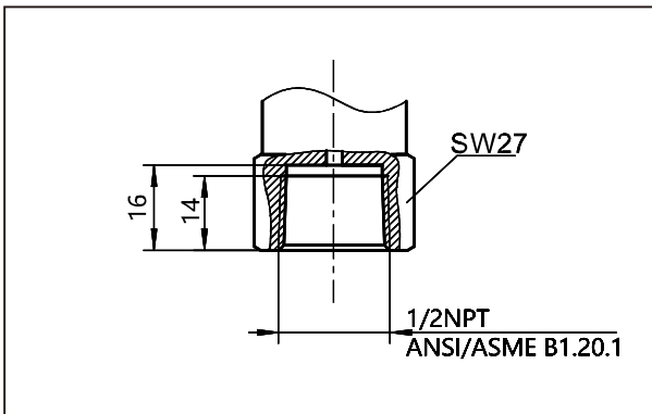
压力导入R03寸法图
