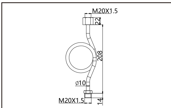
热交换接続部品N1寸法图
