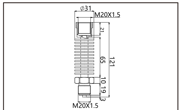
热交换接続部品N2寸法图
