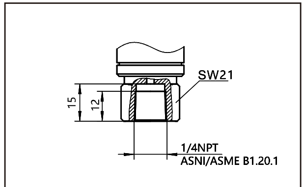
压力导入R04寸法图
