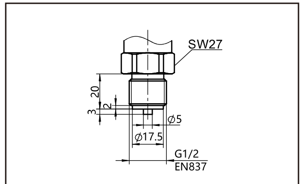
压力导入G01寸法图
