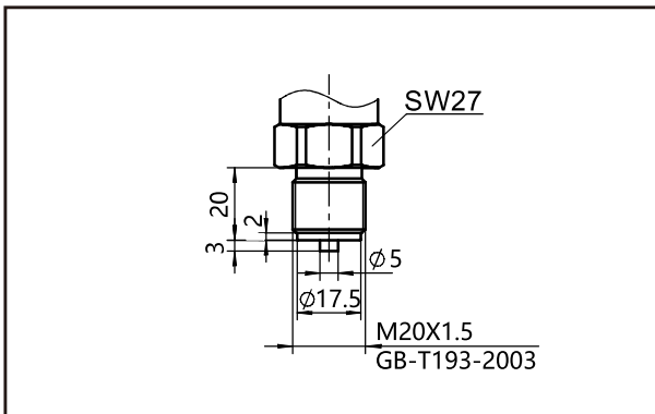
压力导入M01寸法图
