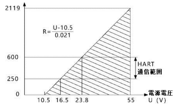
图 1 電源及び負荷条件
